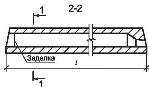
Рисунок 1 — Сечения плит типов 1ПК, 2ПК, 3ПК, 5ПК, 6ПК, 7ПК
