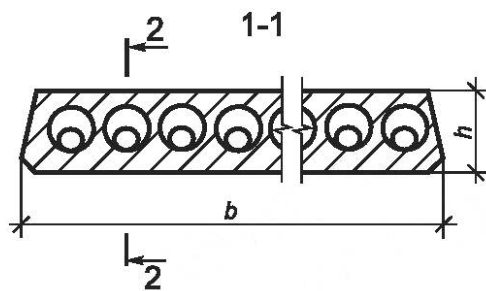
а) Типы 1ПК, 2ПК, 3ПК, 5ПК, 6ПК, 7ПК
