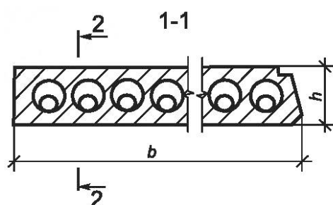
б) Типы 1ПКТ, 2ПКТ, 3ПКТ
