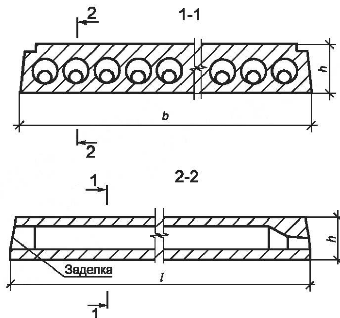
Рисунок 2 — Сечения плиты типа 4ПК
