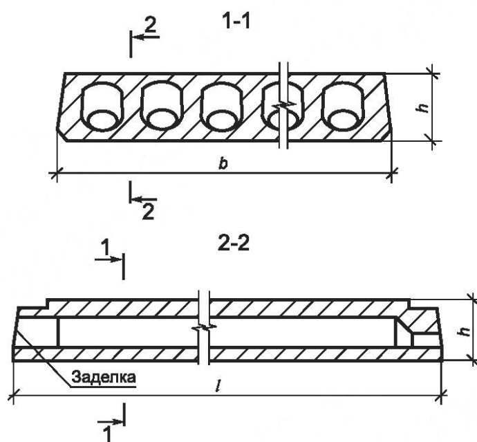
Рисунок 3 — Сечения плиты типа ПГ
