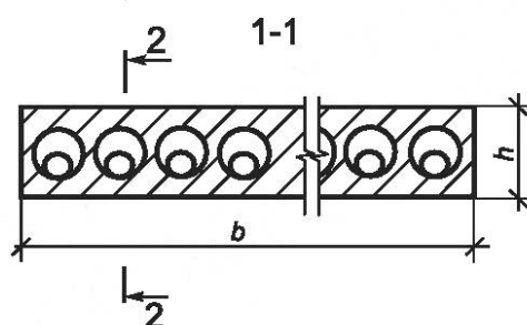
в) Типы 1ПКК, 2ПКК, 3ПКК
