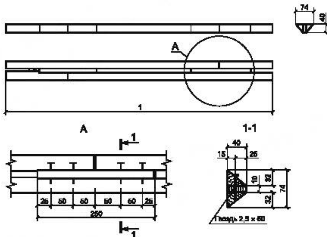
Рисунок А.1 — Пример стыкования брусков обвязки
