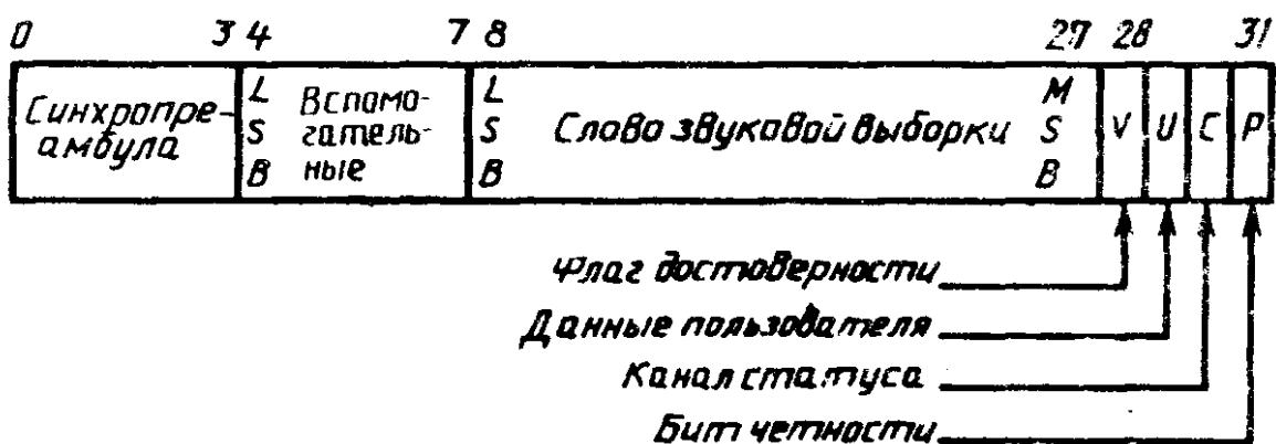
Формат субкадра
