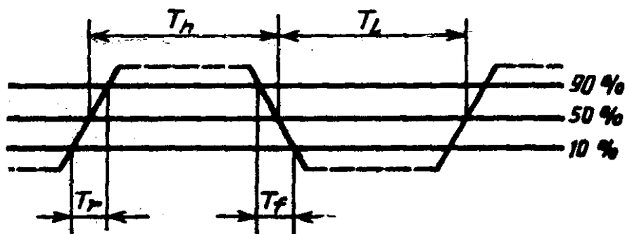
Времена нарастания и спада
