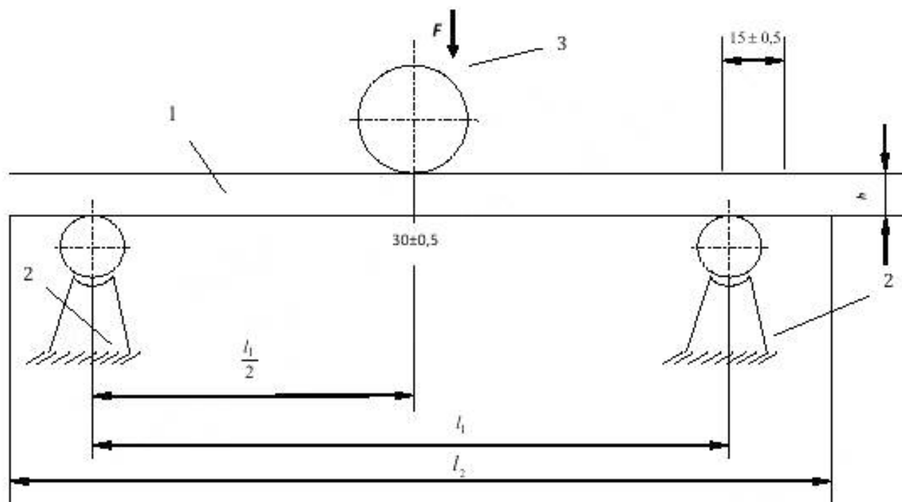
Рисунок 1 – Схема испытания образцов
