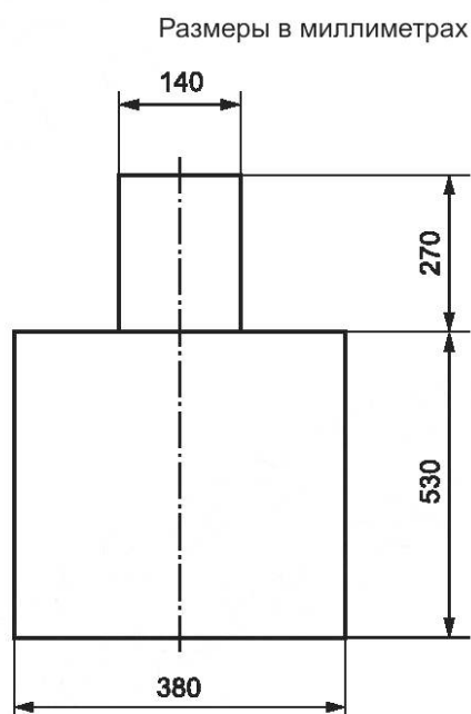
Рисунок А.1 — Испытательный объект, имитирующий сидящего человека
