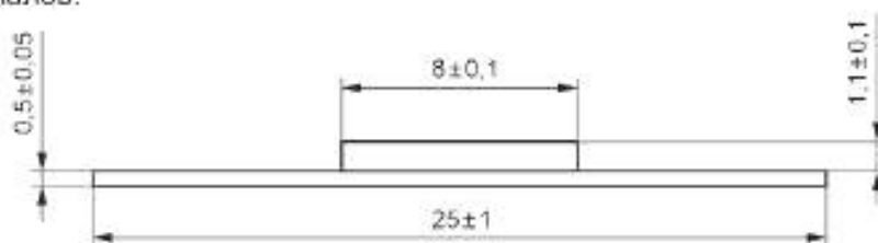
Рисунок 1 — Форма образца для испытаний
