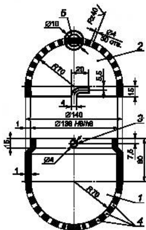
1 — нижняя часть контейнера, 2 — крышка; 3 — две шпильки диаметром 4 мм и длиной 20 мм; 4 — отверстия диаметром 4 мм с шагом 8 мм на нижней части контейнера и крышке; 5 — кольцо диаметром 10 мм
