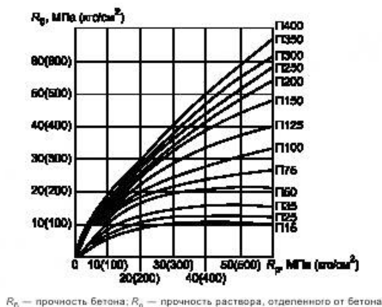
Рисунок 10 — Номограмма для определения марочной прочности крупного заполнителя
