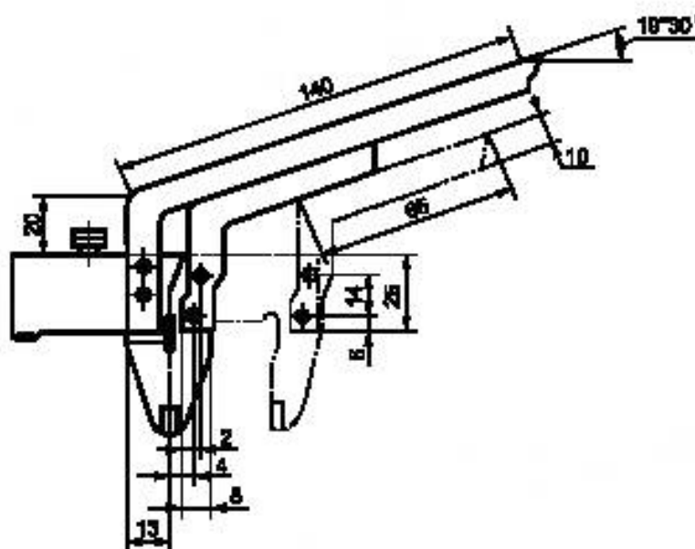
Рисунок 6 — Передвижной шаблон
