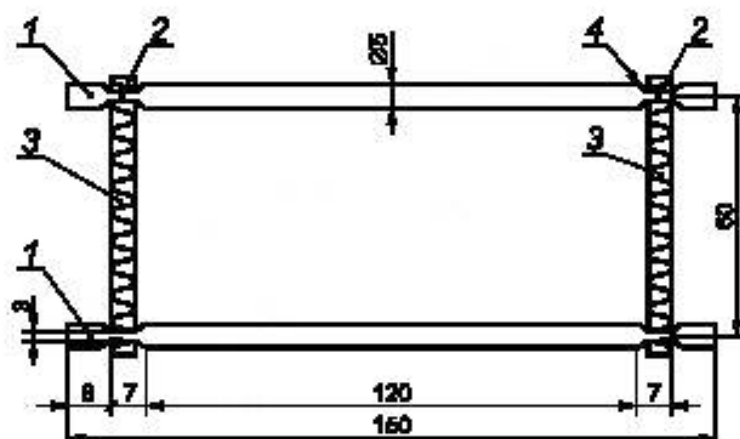
1 — металлические стержни диаметром 5 мм; 2 — места расточки стержней до диаметра 3 мм; 3 — резинка-поддержка (или стальная пружина); 4 — места прошивки резинки
