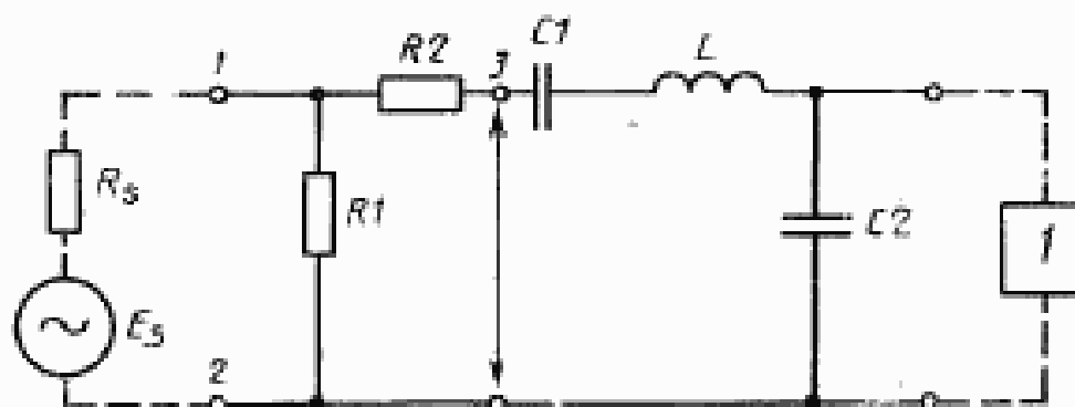
1 — радиоприемник; E_s — ЭДС источника сигнала; R_s — номинальное выходное сопротивление источника сигнала; R_1 , R_2 , C_1 , C_2 , L — резисторы, конденсаторы и катушка индуктивности соответственно
