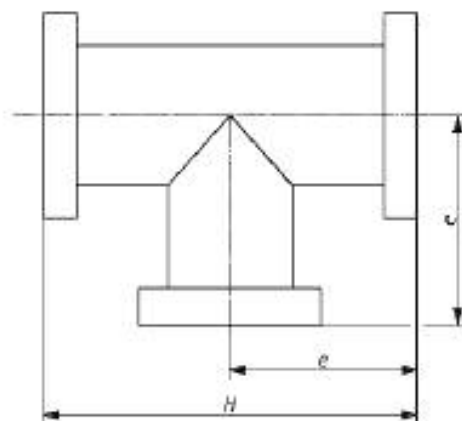
Рисунок 2 – Тройник
