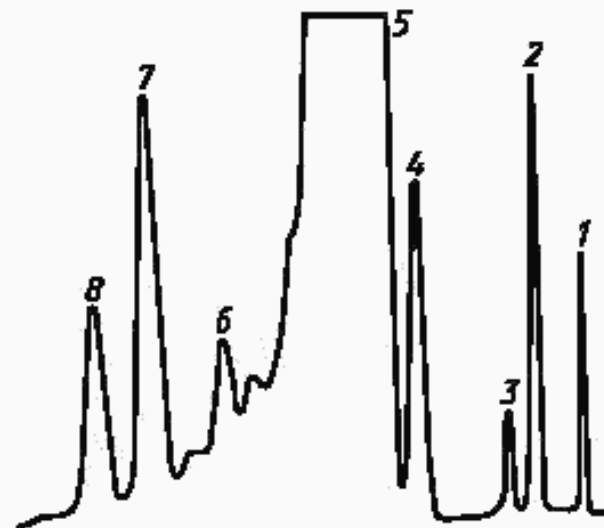
Типовая хроматограмма
