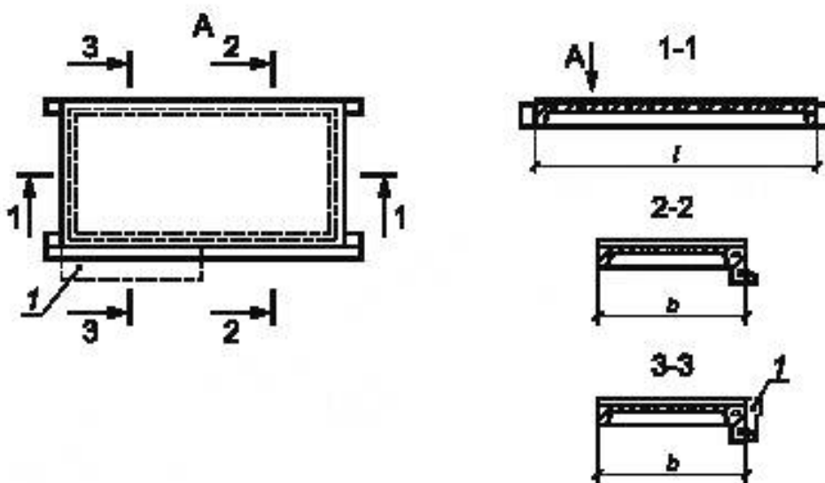
Рисунок 6 — Площадка типа ЛПФ
