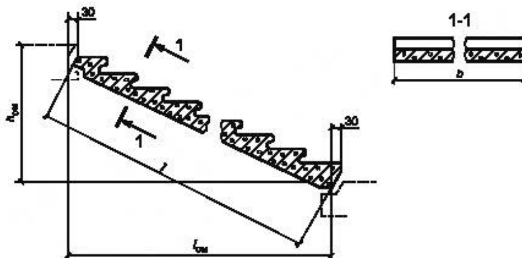
Рисунок 1 — Марш типа ЛМ
