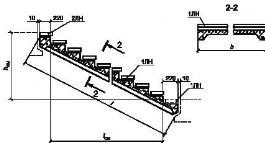
Рисунок 2 — Марш типа ЛМФ
