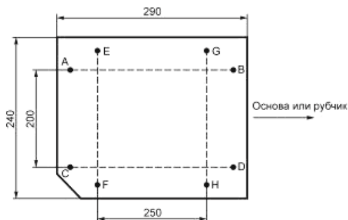
Рисунок 1 — Образцы для испытаний
