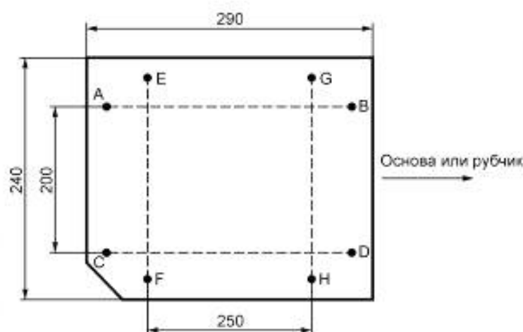
Рисунок 1 — Образцы для испытаний
