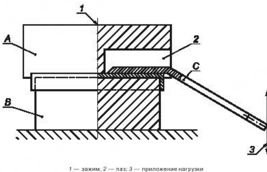
Рисунок 4 — Устройство для зажимания корпуса зеркала
