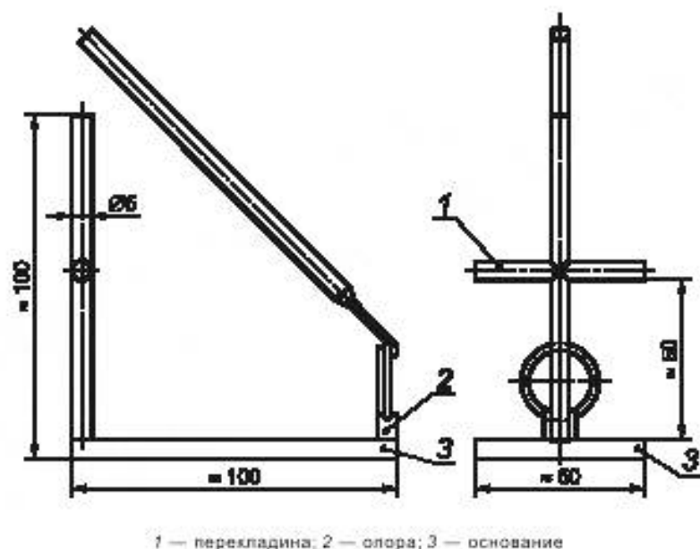
Рисунок 3 — Устройство для проверки искажений (см. 4.3.4)
