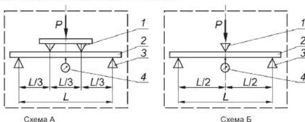
Рисунок 1 – Схема установки для определения модуля упругости
