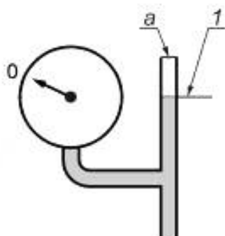
1 — эталонная плоскость манометра; а — открыто в атмосферу
