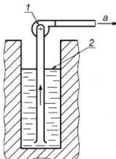
Рисунок В.1 — Кавитационные испытания.
