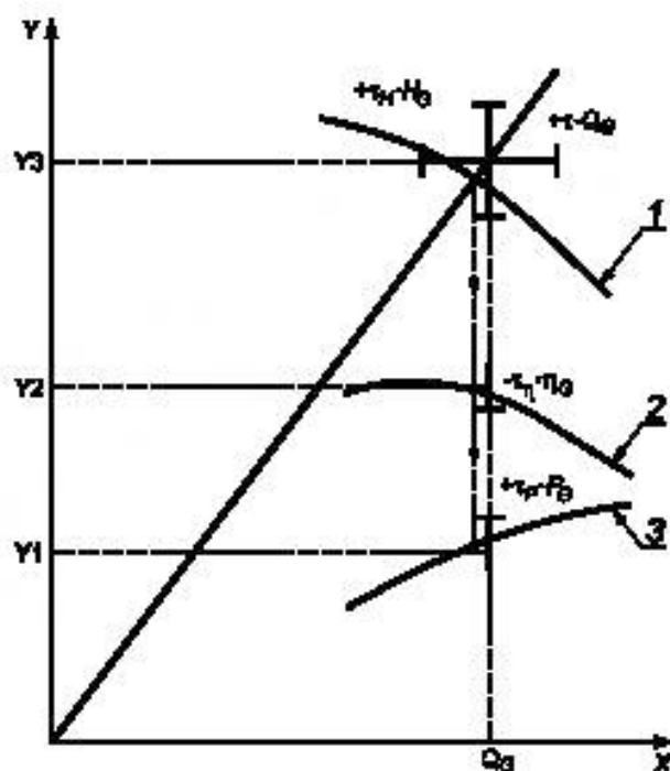
Рисунок 6 — Поле допуска для классов точности 1В, 2В и 3В
