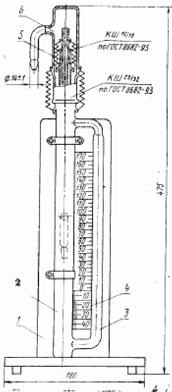
1—подставка; 2—корпус реометра; 3—на- нометрическая трубка; 4—шкала; 5—ка- пилляр; 6—колпачок
