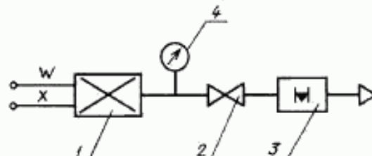
Схема для определения максимальной отдачи воздуха
