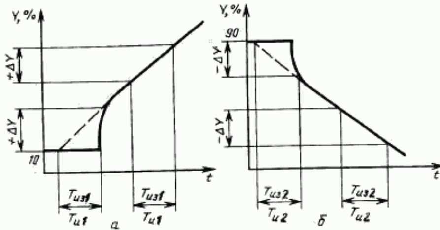
График для определения времени изохрома и интегрирования
