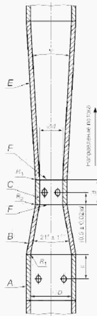
E — диффузор; C — горловина; B — сужающаяся коническая часть; A — входной цилиндрический участок; F — плоскости соединения элементов трубы Вентури; s — см. 5.4.7
