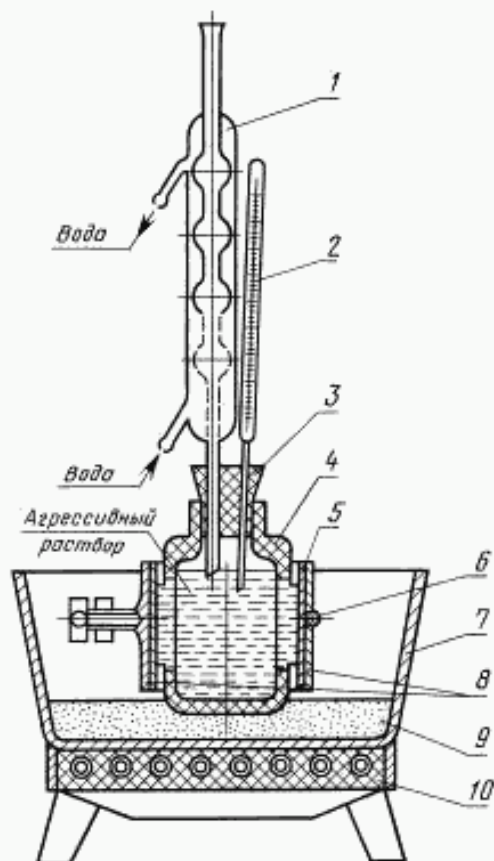
1 — холодильник; 2 — термометр; 3 — пробка; 4 — фарфоровый сосуд или сосуд из нержавеющей стали; 5 — прокладка; 6 — зажим; 7 — ванночка; 8 — образец; 9 — песок; 10 — электрическая плита
