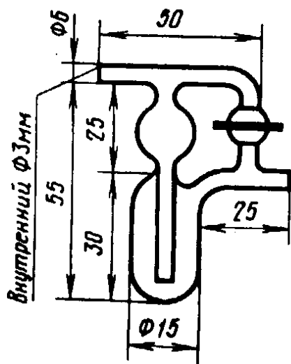
Склянка Дрекселя с краном
