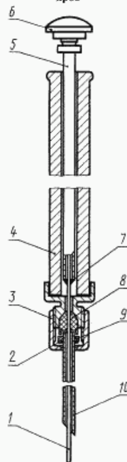
1 — поршень; 2 — прокладка; 3 — гайка коническая; 4 — корпус МШ-1; 5 — шток МШ-1; 6 — головка МШ-1; 7 — пайка; 8 — сальник; 9 — фланец иглы; 10 — игла
