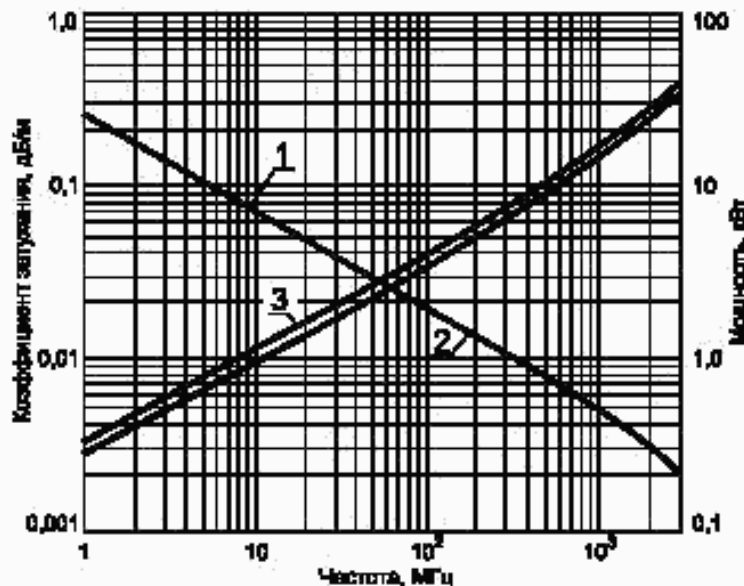
Частотные зависимости
