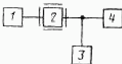
1 — высокочастотный генератор сигналов; 2 — приемник; 3 — испытательная нагрузка приемника; 4 — низкочастотный вольтметр.
