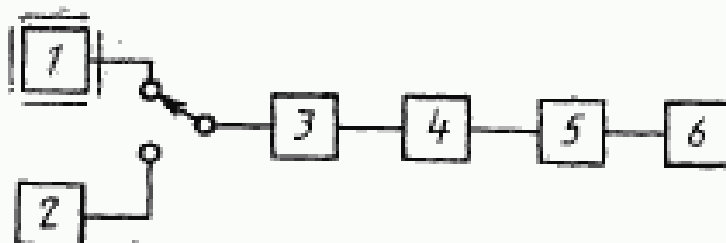
1 — передатчик; 2 — высокочастотный генератор сигналов; 3 — нагрузочная нагрузка передатчика; 4 — аттенюатор; 5 — режекторный фильтр; 6 — измерительный приемник (табл. 6, п. 11)
