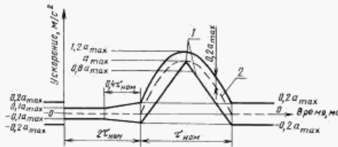
1 — пределы отклонений; 2 — номинальный пробег; a_{max} — пиковое ускорение удара; \tau_{ном} — длительность ударного импульса
