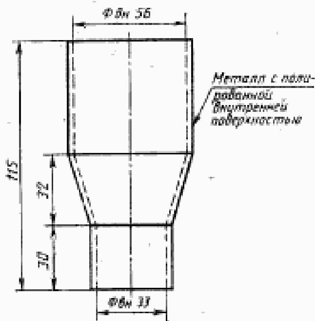
Воронка для определения насыпной плотности
