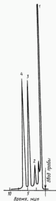
Хроматограмма фенолоанилиноформальдегидных смол
