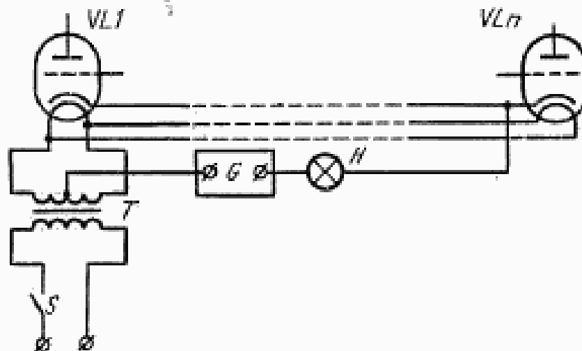
VL1, VL2—испытываемые лампы; T—накальный трансформатор; S—прерыватель напряжения накала; G—источник питания участка катод-подогреватель; H—сигнальная лампа
