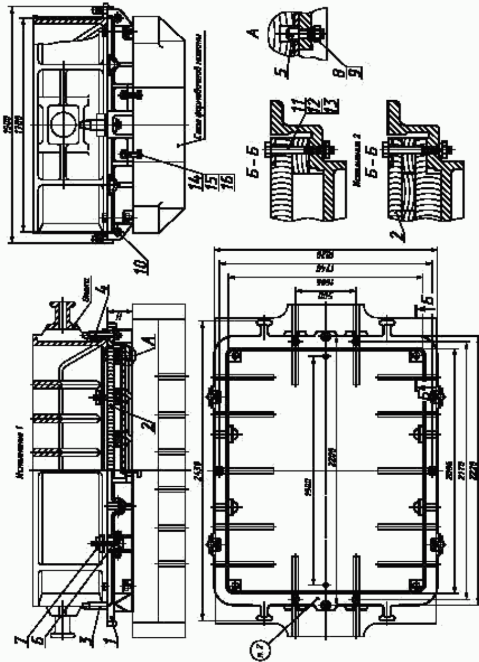
1 — рама по табл. 1; 2 — вкладыш по табл. 1; 3 — штырь центральный 0290-2508 по ГОСТ 20122 (кол. 1); 4 — штырь направляющий 0290-2558 по ГОСТ 20123 (кол. 1); 5 — штырь контрольный 0298-0122 по ГОСТ 20172 (кол. 2); 6 — штырь откидной 0290-2032 по ГОСТ 20128 (кол. 4); 7 — клин крепежный 0292-0615 по ГОСТ 19391 (кол. 4); 8 — гайка М12—6Н.6.05 по ГОСТ 5927 (кол. 2); 9 — шайба 12.65Г.05 по ГОСТ 6402 (кол. 2); 10 — болт М20—6g×120.66.05 по ГОСТ 7808 (кол. 4); 11 — болт М16—6g×140.66.05 по ГОСТ 7808 (кол. 4); 12 — гайка М16—6Н.6.05 по ГОСТ 5927 (кол. 4); 13 — шайба 16.65Г.05 по ГОСТ 6402 (кол. 4); 14 — болт М20—6g×95.66.05 по ГОСТ 7808 (кол. 6); 15 — гайка М20—6Н.6.05 по ГОСТ 5927 (кол. 12); 16 — шайба 20.65Г.05 по ГОСТ 6402 (кол. 8)
