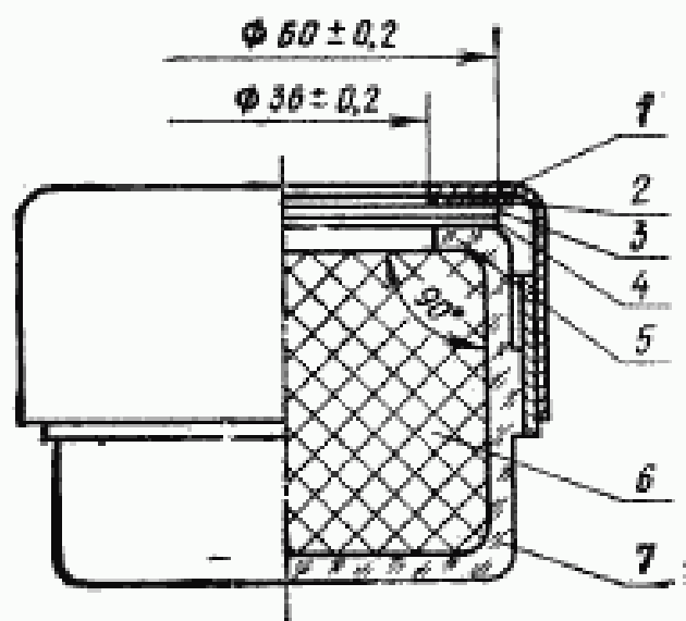
1—крышка; 2—резиновая прокладка; 3—образец; 4—влагонепроницаемая пленка; 5—заплечики; 6—вкладыш из пенополиуретана; 7—стеклянный стаканчик.
