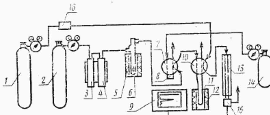
Установка для определения содержания углерода
