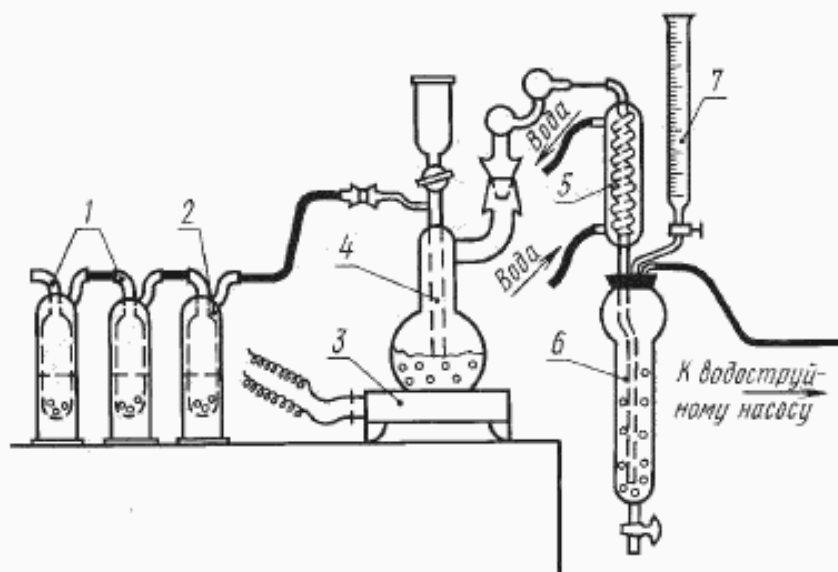
1 — склянка-ловушка с серной кислотой; 2 — склянка-ловушка с водой; 3 — электролитка; 4 — дистилляционная колба типа Кьельдаля из термостойкого стекла вместимостью 500 см 3 с притертой пробкой, снабженной каплевой воронкой с краном; 5 — холодильник; 6 — сосуд для улавливания аммиака; 7 — микробюретка
