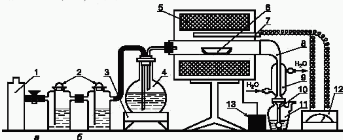
1 — баллон с газом; 2 — очистительные склянки; а — раствор \text{KMnO}_4 в растворе \text{NaOH} , б — дистиллированная вода; 3 — электроплитка; 4 — парообразователь; 5 — трубчатая электропечь сопротивления; 6 — лодочка кварцевая; 7 — платино-платинородиевая термопара; 8 — кварцевая трубка; 9 — холодильник; 10 — отводная трубка; 11 — колба-приемник; 12 — милливольтметр; 13 — трансформатор напряжения для регулирования температуры печи
