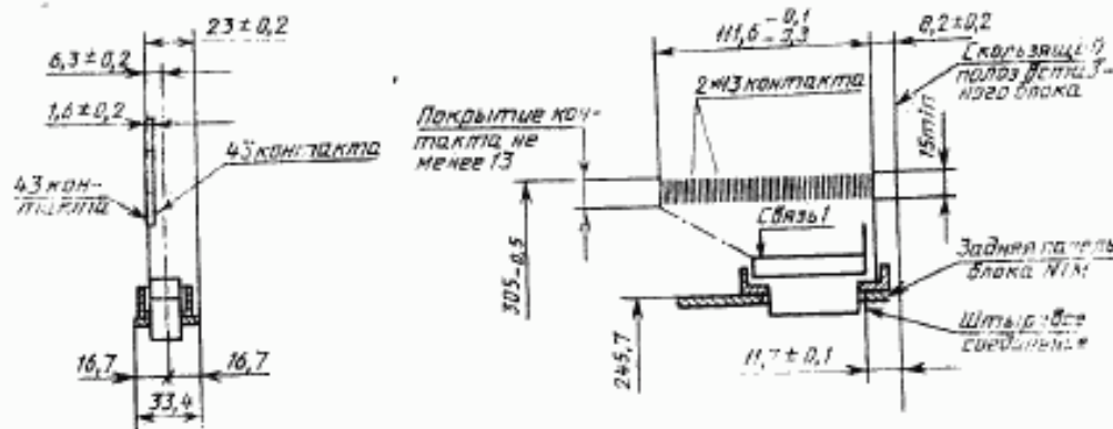
Рисунок 7 — Адаптер для блоков NIM
