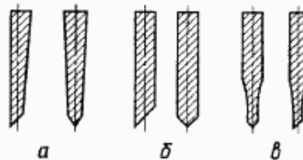
a — клиновидное сечение; b — прямоугольное сечение; v — прямоугольное сечение с фаской (ширина фаски — 5 мм и более)
