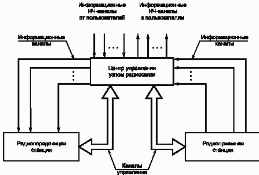
Рисунок А.1 — Упрощенная структурная схема УРС
