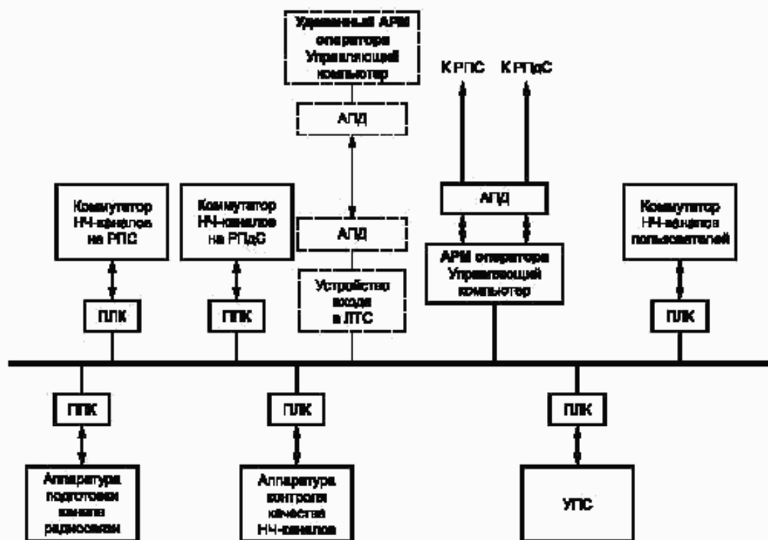
Рисунок 1 — Структурная схема ЛТС на уровне ЦУ
