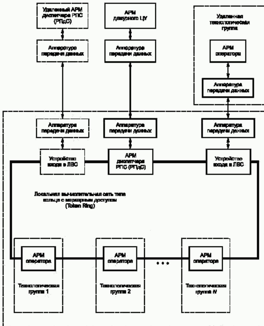
Рисунок 2 — Структурная схема системы управления на уровне РПД (РПС) для ЛВС типа кольца с маркерным доступом
