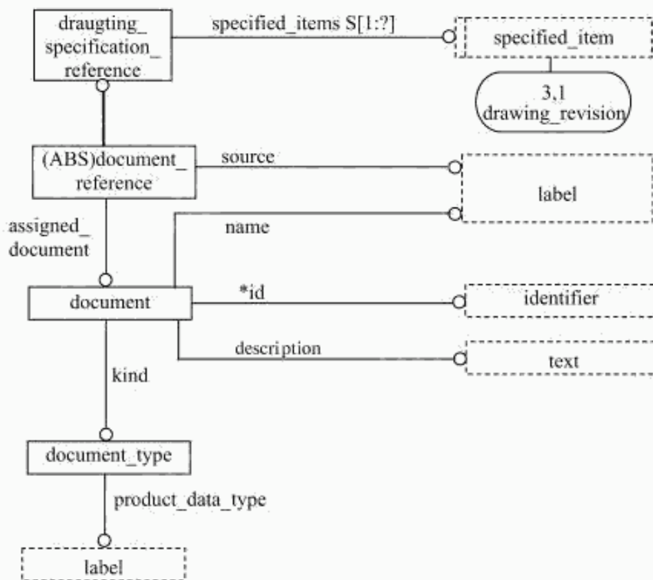
Рисунок С.7 — Расширенный листинг ПИК — EXPRESS-G диаграмма 7 из 14
