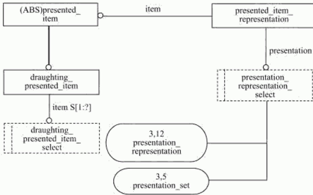
Рисунок С.14 — Расширенный листинг ПИК — EXPRESS-G диаграмма 14 из 14
