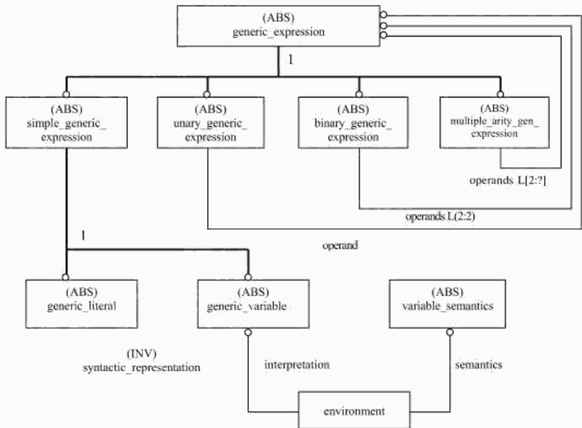
Рисунок С.1 — ISO13584_generic_expressions_schema — EXPRESS-G диаграмма.1 из 1
