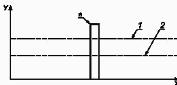
X — время; Y — сигнал датчика фазы; 1 — уровень срабатывания 1; 2 — уровень срабатывания 2; a — один и тот же момент срабатывания по уровням 1 и 2
