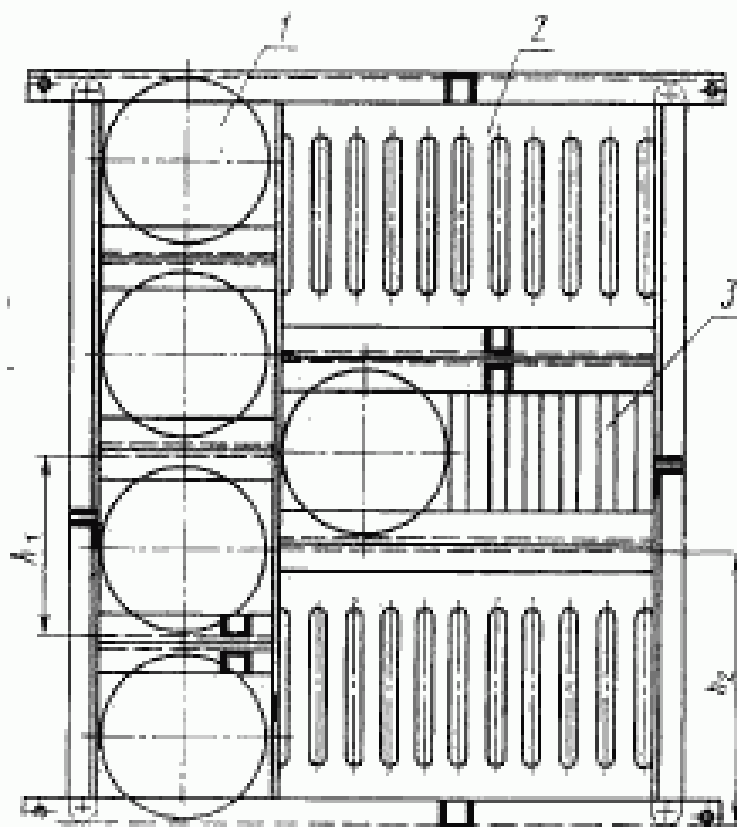
1 — образец в форме диска; 2 — образцы в форме дощечки; 3 — образец в форме бруска; A_1 — высота рамки для образца 1; A_2 — высота рамки для образца 2
