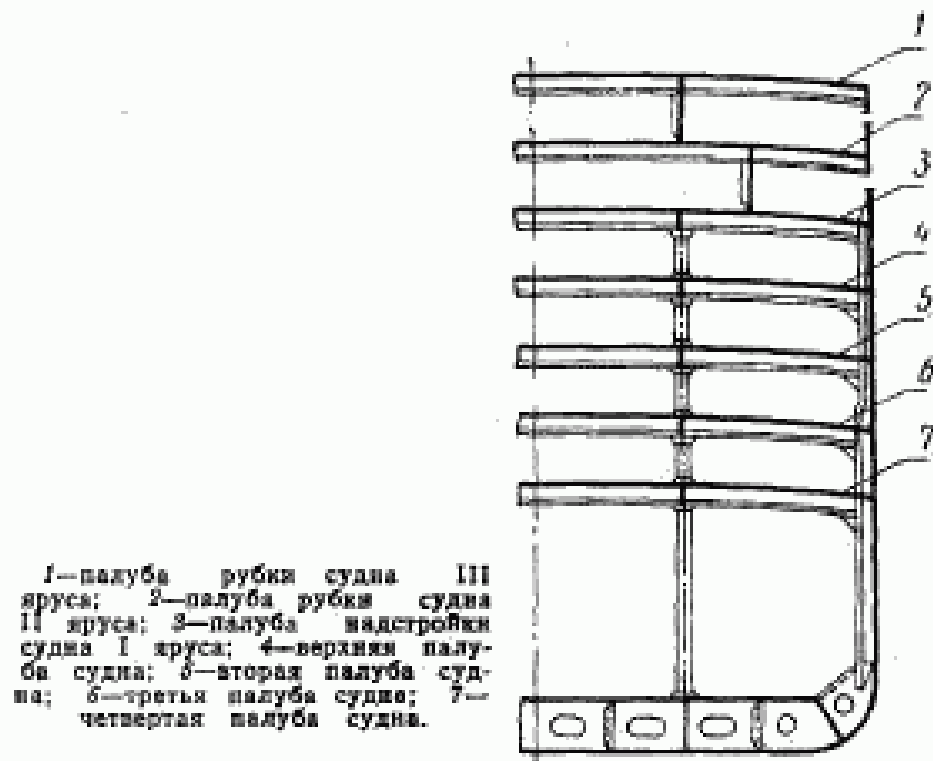
Черт. 1 Схема расположения палуб на судне
