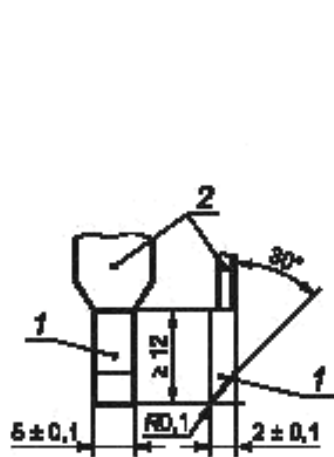
1 — платиновый электрод; 2 — медный удлинитель
