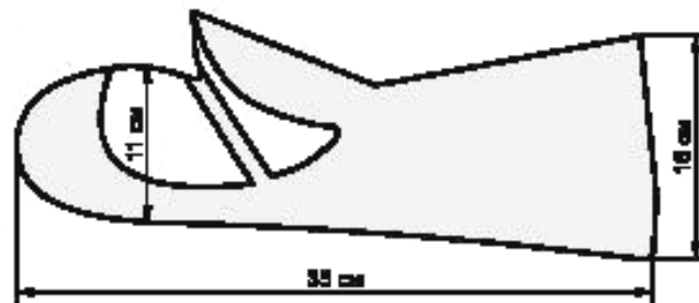
Рисунок 2 — Внутренние минимальные размеры ЗАЩИТНЫХ РУКАВИЦ
