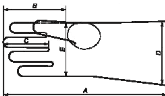
Рисунок 1 — Внутренние размеры ЗАЩИТНЫХ ПЕРЧАТОК
