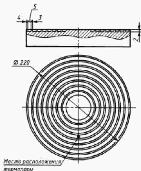
Рисунок В.1— Внешний вид рабочей поверхности электроплиты
